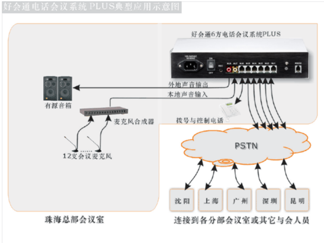
好会通 PLUS 系统采用专业麦克风应用方案拓扑图
